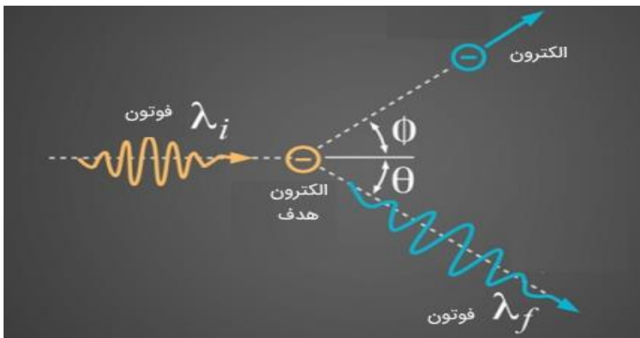
شکل ۸: اشعه گاما (Yousifi, 2022)
