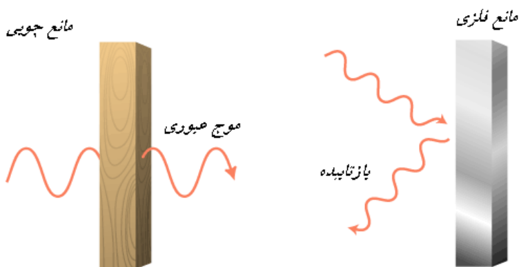
شکل ۲: بیان‌کننده امواج رادیویی (Vecchia, 2007)
