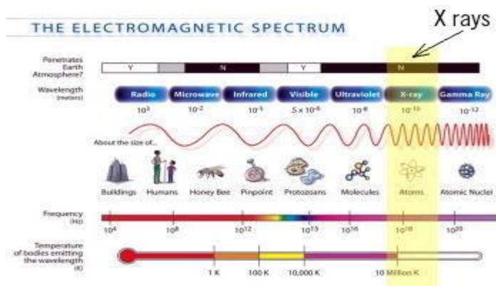
شکل ۵: اشعه ایکس (Vecchia, 2007)
