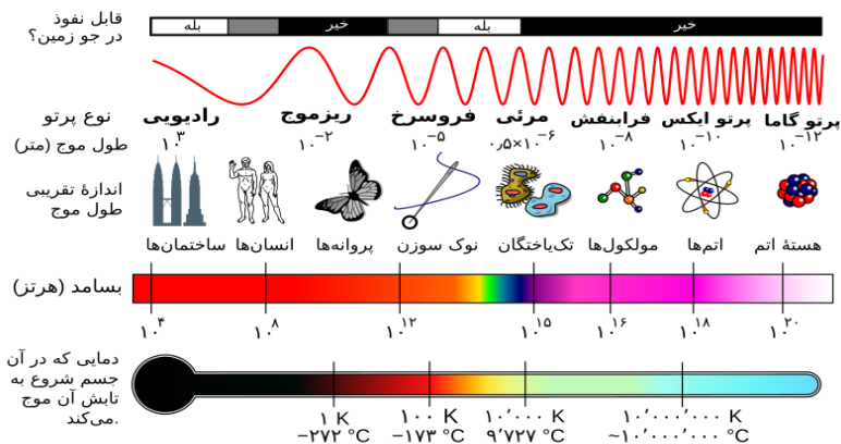
شکل 1: طیف امواج الکترومغناطیسی (Funk, 2006)
